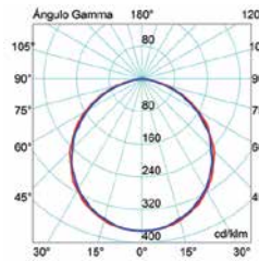
LED-18 Redondo (Iluminación) 71496 / 71498
