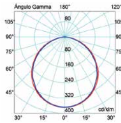
LED-18 Cuadrado (Iluminación) 71497 / 71499
