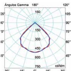
LED-18 Cuadrado (Señalización) 71497 / 71499
